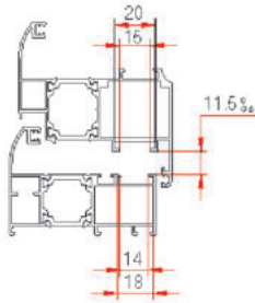
Uygulanabilir Kesit Detayları
